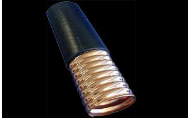
Guía de onda elíptica estándar, 5.6–6.425 GHz, black PE jacket
