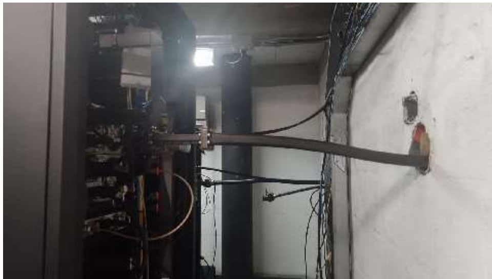
Detalle salida de Guía de Onda desde el cuarto de equipos del Telepuerto
